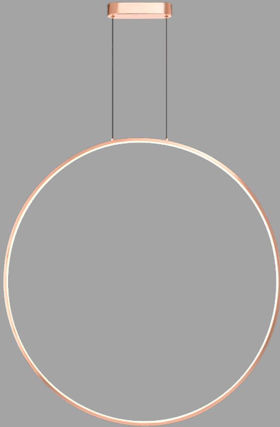
♠ WIN 20141 68900 Ø800 W15 線長 1000mm / LED 27W 3000K / 鋼材電鍍
