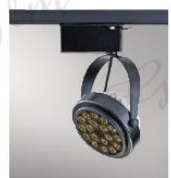
GLM-2644A 2300 L65mm W140mm H220mm 附OSRAM LED 18珠 22W 3000K/4000K/5700K、防眩光鍍黑網 鋁、鍍材加工成型、粉體烤漆
