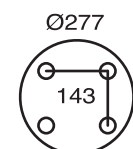
壁座 孔Ø4 附一字活動板
