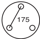
底座Ø233 孔Ø14
