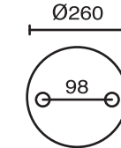
壁座 孔Ø5 附一字活動板
