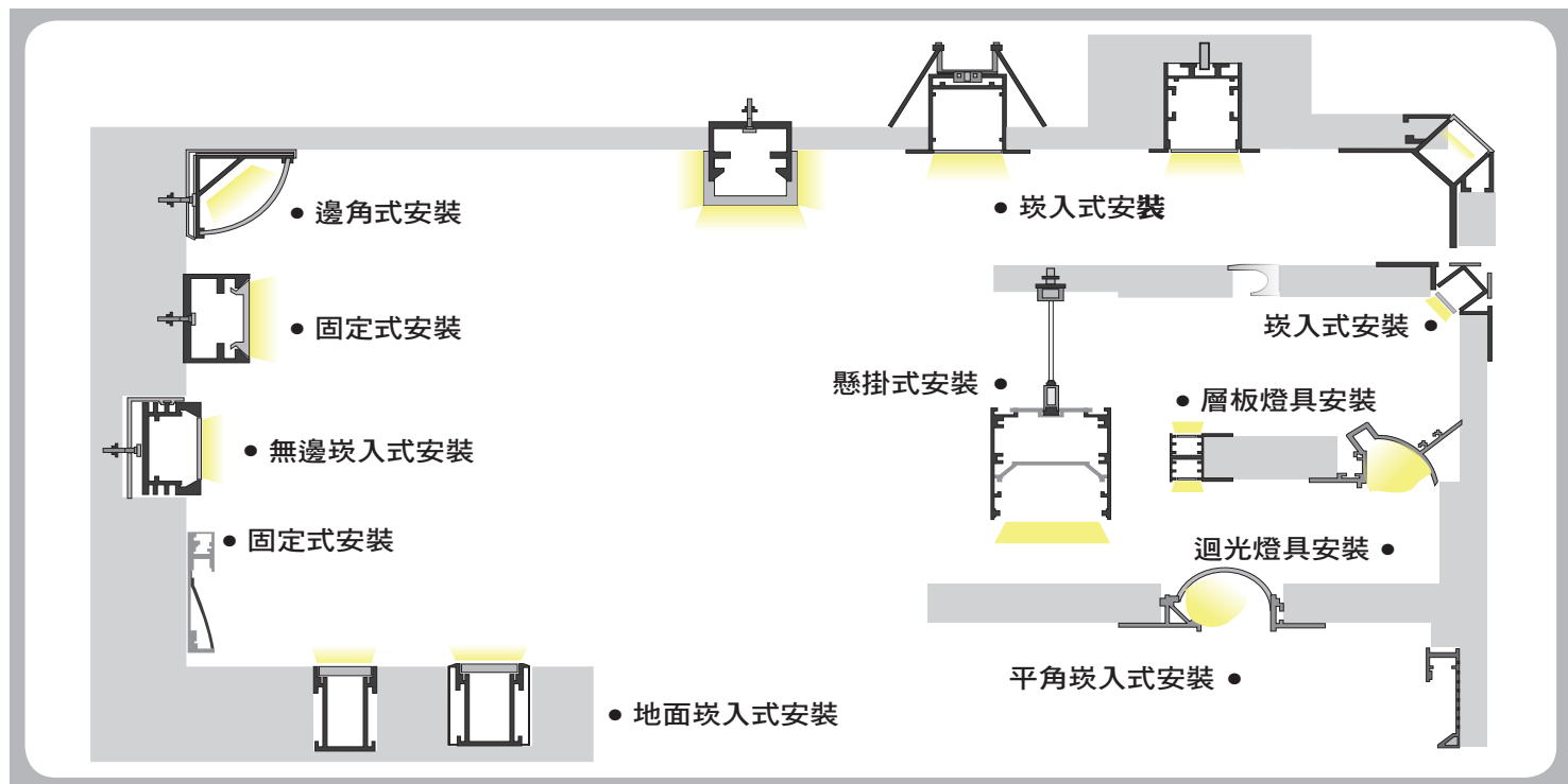
鋁條多種安裝方式圖
