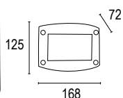
預埋盒尺寸: W160 H96 D75
