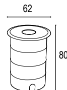
預埋盒尺寸: W48 H90
