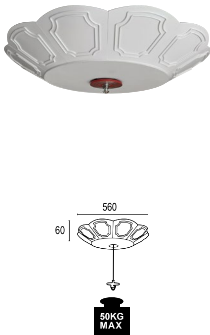
FL-7001-2 62000 Ø560 H60 mm 載重 50 公斤 配置 4 米鋼線 載重物：15~50 公斤
