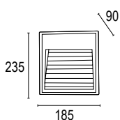
預埋盒尺寸: W180 H225 D96
