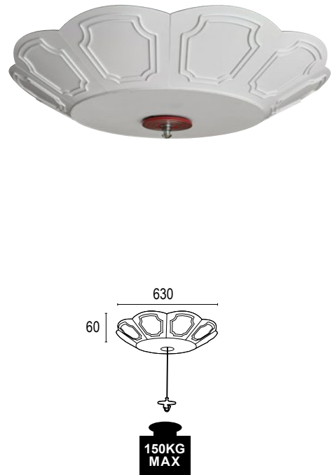
FL-7001-3 107000 Ø630 H60 mm 載重 150 公斤 配置 6 米鋼線 載重物：50~150 公斤
