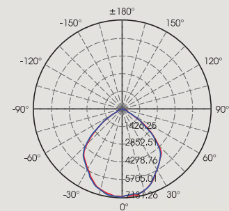
【配光曲線】
