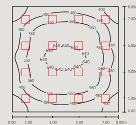
【模擬照度圖】
