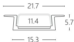
(尺寸圖)
