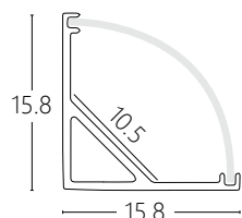
(尺寸圖)
