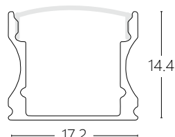
(尺寸圖)
