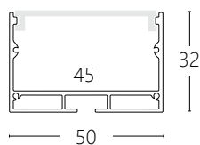
(尺寸圖)
