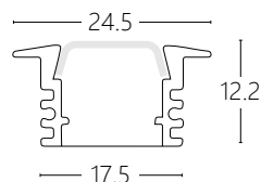
(尺寸圖)
