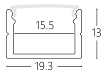
(尺寸圖)
