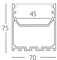
(尺寸圖)
