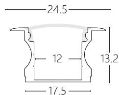
(尺寸圖)
