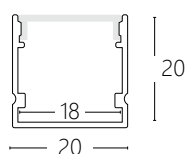
(尺寸圖)
