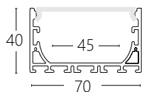
(尺寸圖)
