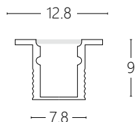
(尺寸圖)
