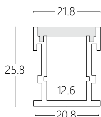
(尺寸圖)
