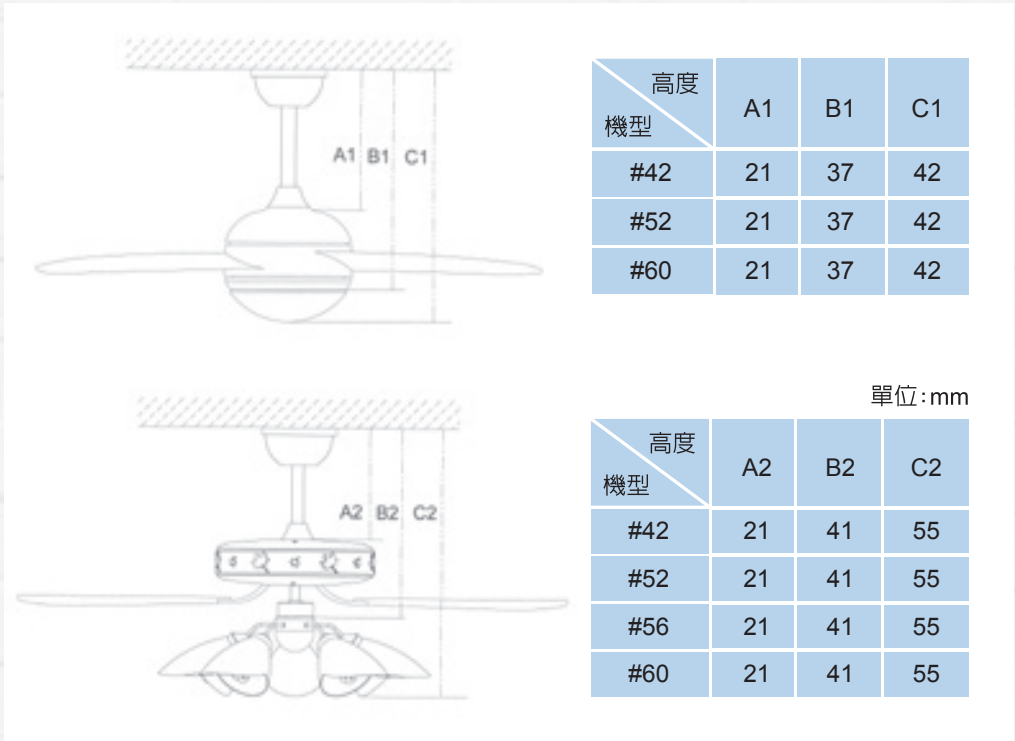
吊扇及燈具組的高度
