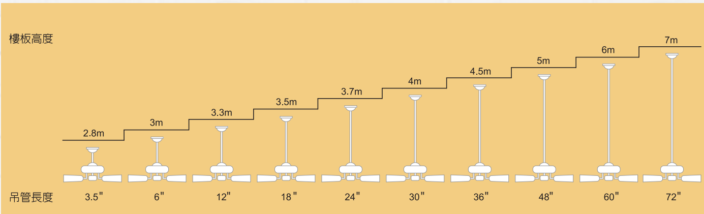
吊扇高度(Ceiling Height)
